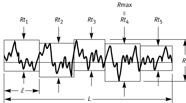
Fig. 1-11 The R_t and R_{max} Parameters
