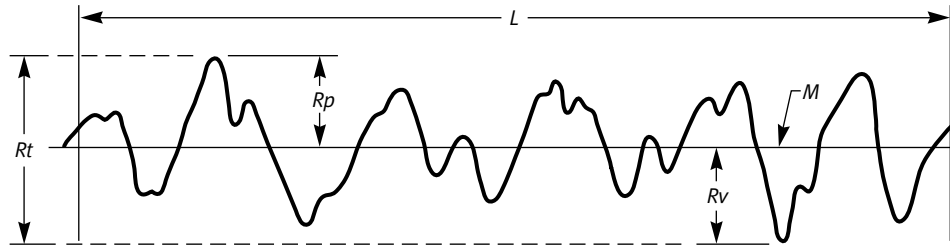
Fig. 1-9 R_t , R_p , and R_v Parameters
