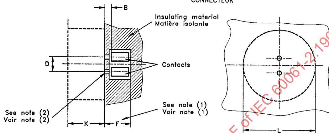
Fig.1 CONNECTOR CONNECTEUR
