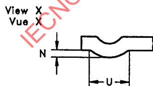
Enlarged detail of retention indent Détail agrandi du bossage d'arrêt
