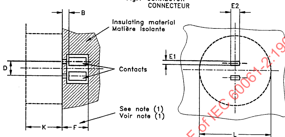
Fig.1 CONNECTOR CONNECTEUR
