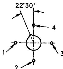
Top view of lampholder Vue de la douille par-dessus
