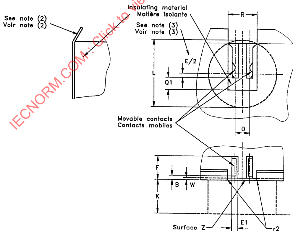
Fig.2 CONTACT ASSEMBLY WITH PARALLEL SLIDE-IN GROOVES BLOC DE CONTACT AVEC RAINURES DE GUIDAGE PARALLELES
