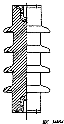
Figure 3 – Support isolant cylindrique à armatures internes
