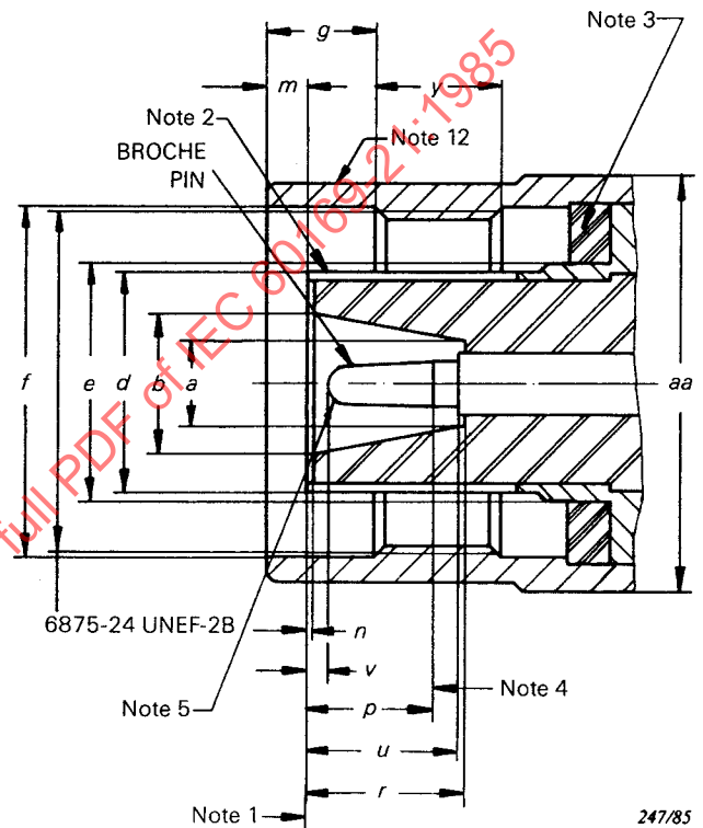
FIG. 2. — Connecteur avec contact central mâle (SC-B). Connector with pin centre contact (SC-B).
