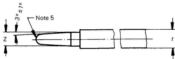
FIG. 3. — Détail du contact mâle. Detail of pin contact.
