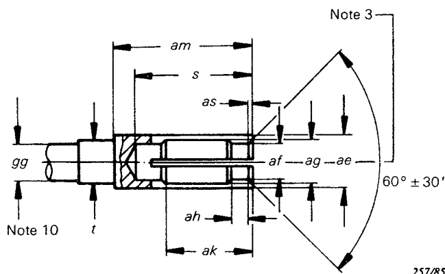
FIG. 11. — Connecteur d'essai de référence avec contact femelle. Standard test connector with socket contact.
