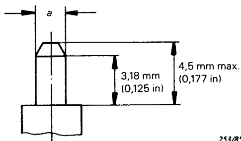
FIG. 8. – Calibre (broche) pour le contact central du connecteur femelle. Gauge (pin) for centre contact of socket connector.
