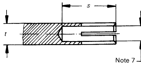
FIG. 6. - Détail du contact femelle. Detail of socket contact.
