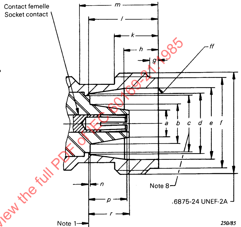
FIG. 5. - Connecteur avec contact central femelle (SC-B). Connector with socket centre contact (SC-B).
