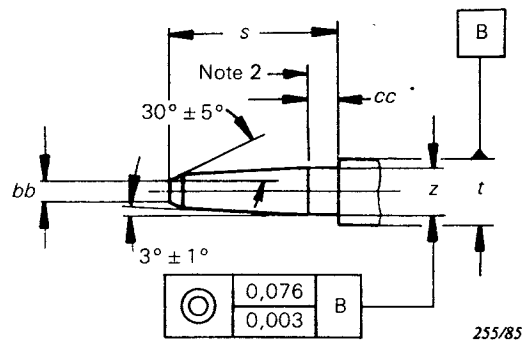
FIG. 10. — Détail du contact mâle. Detail of pin contact.
