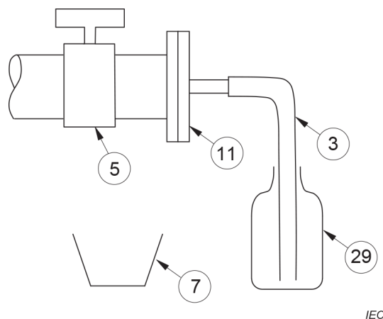
a) Exemple d'échantillonnage en flacon
