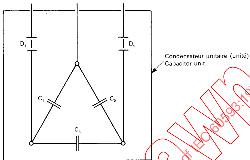
FIG. 1. — Schéma d'une unité triphasée, connectée en triangle, avec deux déconnecteurs à surpression ( D_1 et D_2 ).
