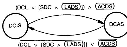
Figure 12 – Diagramme d'états de la fonction libération d'appareil
