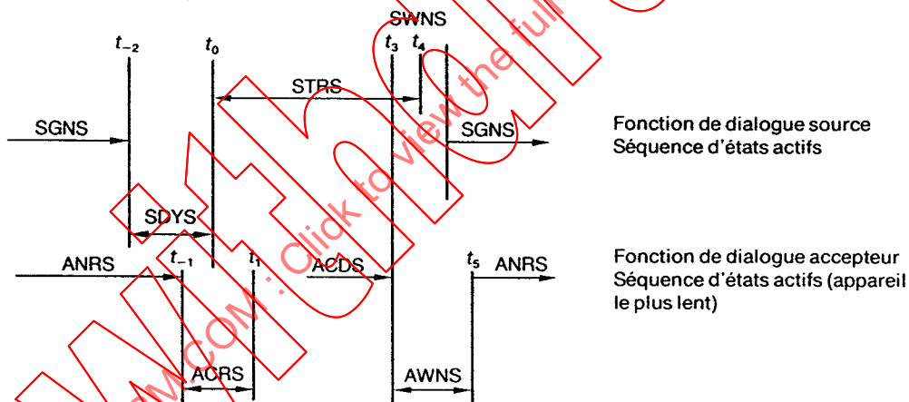
Figure B.1 – Séquence de temps pour un parleur et plusieurs écouteurs utilisant le procédé de dialogue
