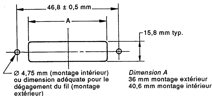
Figure 18 – Echancrure dans le panneau pour recevoir le connecteur
