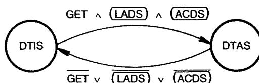
Figure 13 – Diagramme d'états de la fonction déclenchement d'appareil
