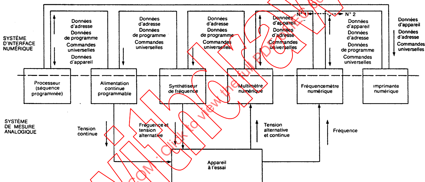
Figure A.1 – Système type d'instrumentation
