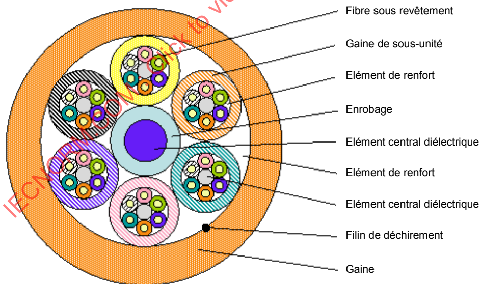
Figure A.2 – Exemple de coupe transversale d'un câble composé de 36 fibres
