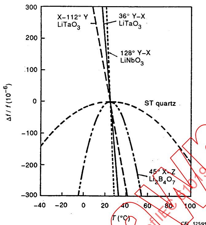
Figure 11 – Caractéristiques température-fréquence pour divers matériaux habituellement utilisés et leurs angles de coupe
