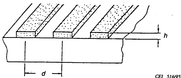
4a- Bandes métalliques ou arêtes diélectriques
