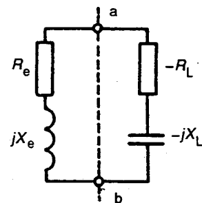
12c - Circuit équivalent
