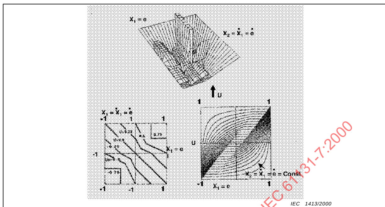
Figure A.12 – Exemples de courbes de caractéristiques de contrôle flou
