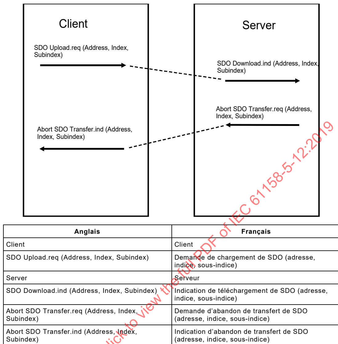
Figure 15 – Séquence d'un seul SDO-Upload qui a échoué
