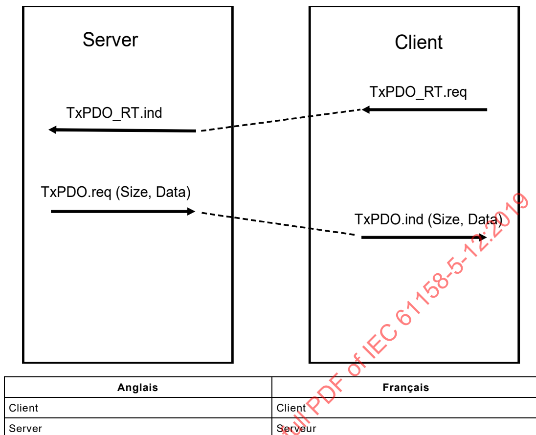
Figure 25 – Séquence "TxPDO remote transmission" (émission distante TxPDO)
