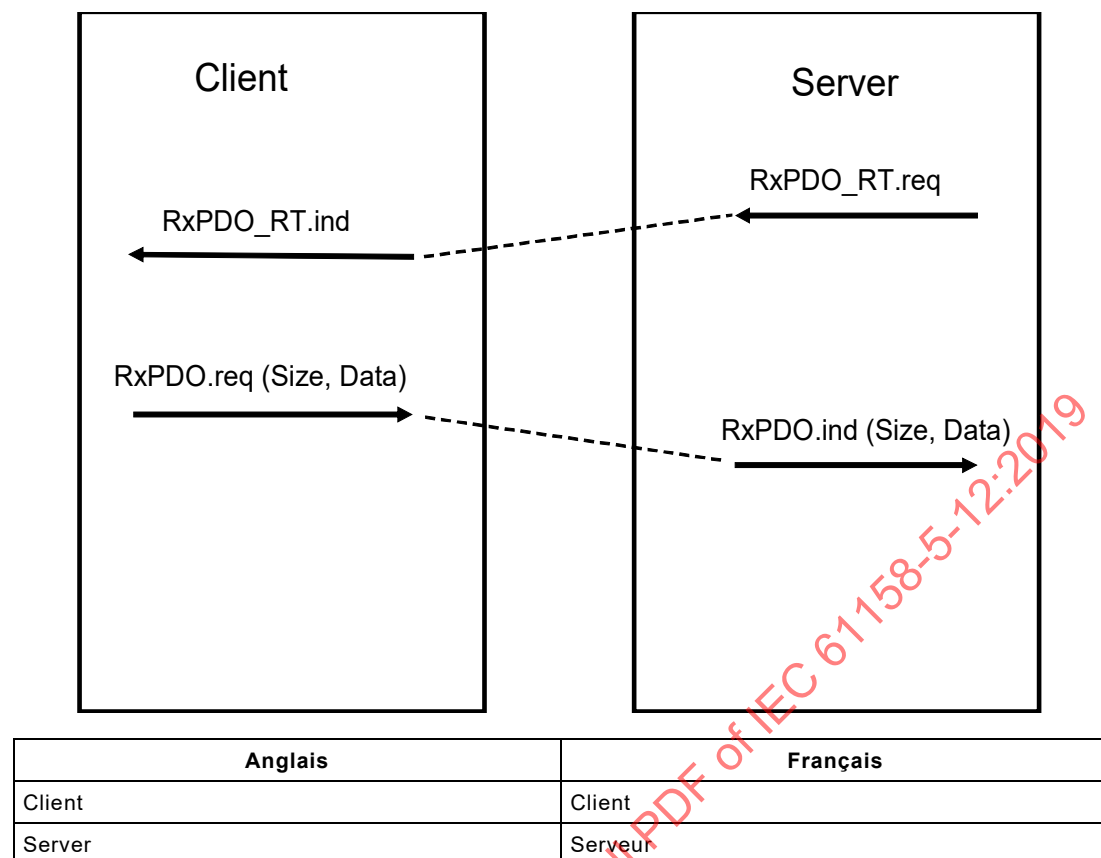
Figure 24 – Séquence "RxPDO remote transmission" (émission distante RxPDO)
