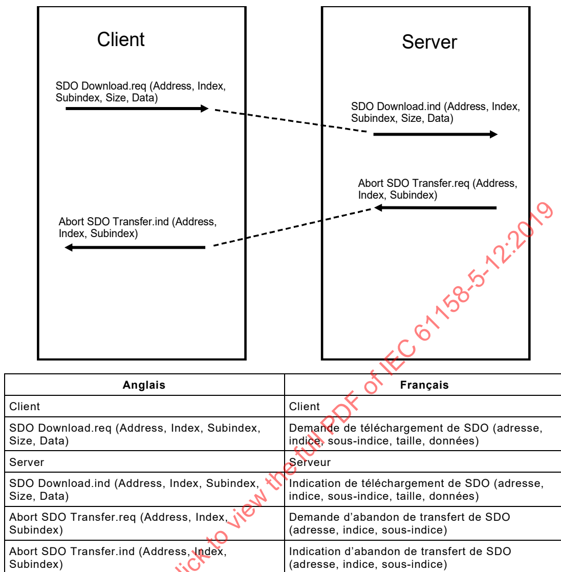
Figure 12 – Séquence d'un seul SDO-Download qui a échoué
