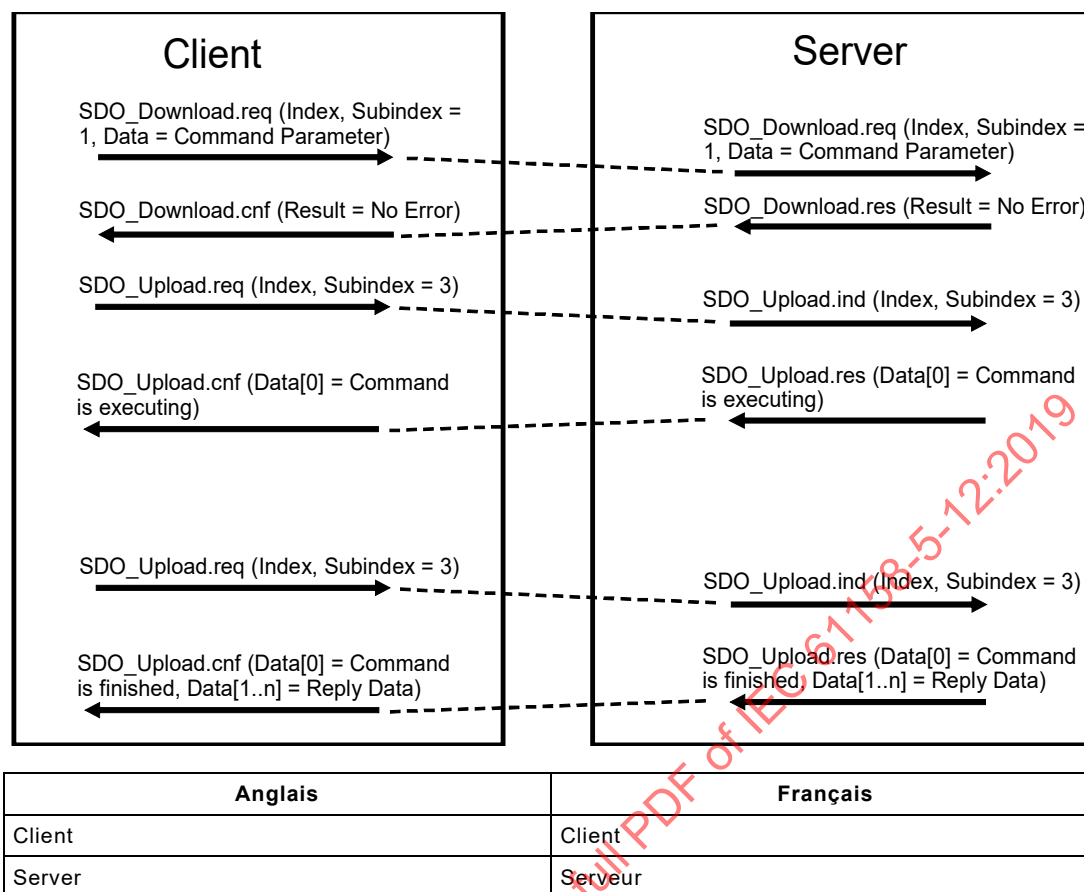
Figure 19 – Séquence de "Command"
