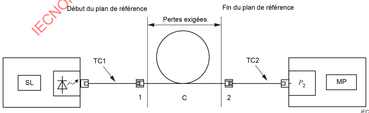
Figure 3 – Plan de référence pour la configuration d'essai A avec la méthode à cordon unique
