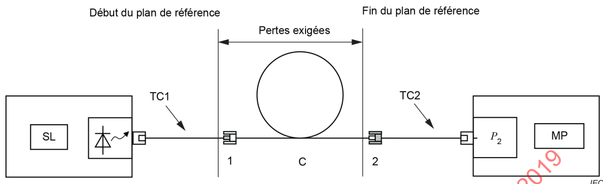
Figure 4 – Plan de référence pour la configuration d'essai B avec la méthode à 3 cordons
