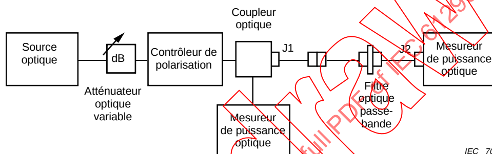
Figure 1b - Mesure des pertes du filtre passe-bande optique et de la jarretière de fibre optique
