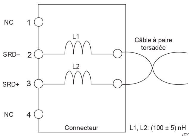
Figure A.7 – Connecteur de câble à bobines d'inductance
