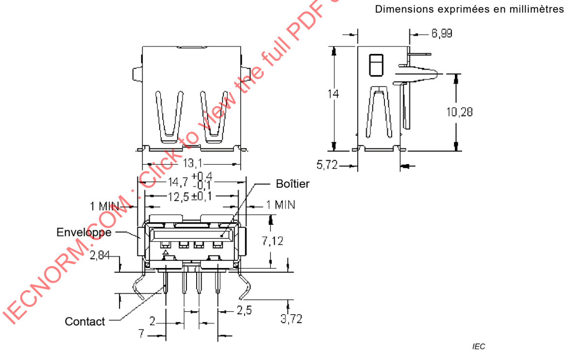
Figure A.4 – Dimensions d'un connecteur de dispositif à un port
