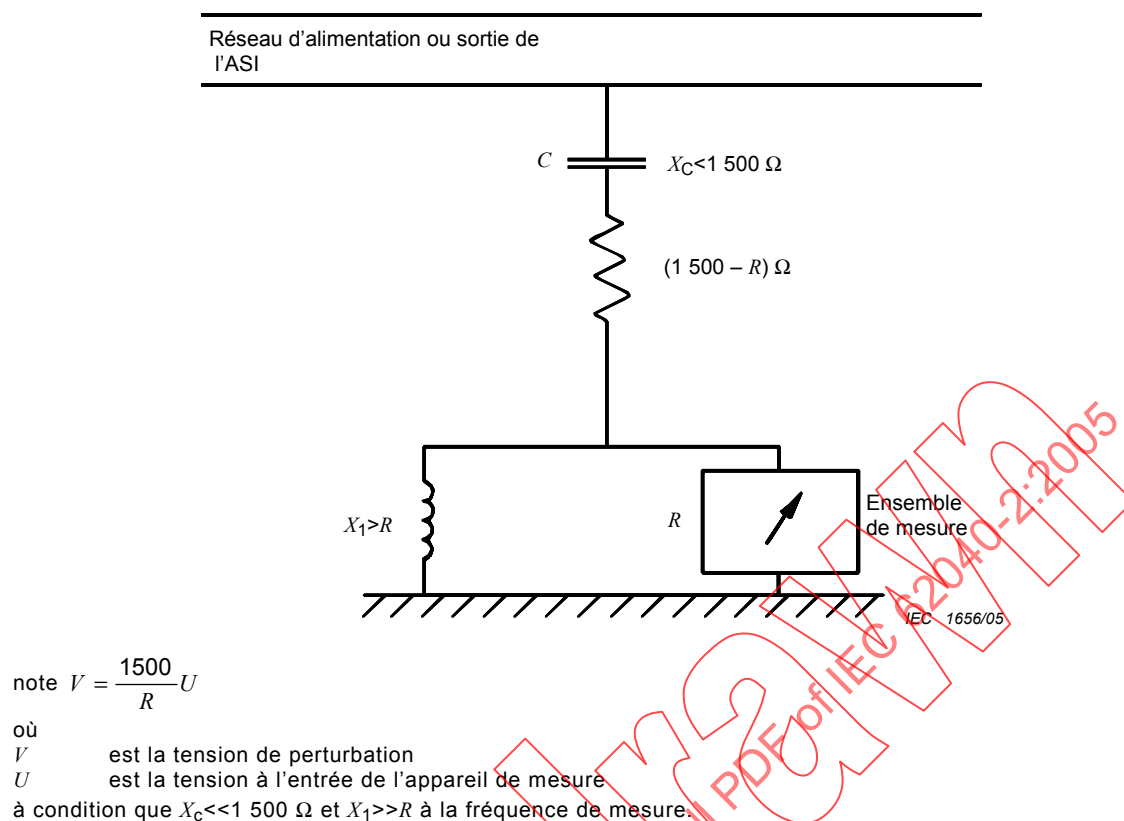
Figure A.1 – Circuit de mesure des tensions perturbatrices sur le réseau d'alimentation ou la sortie de l'ASI
