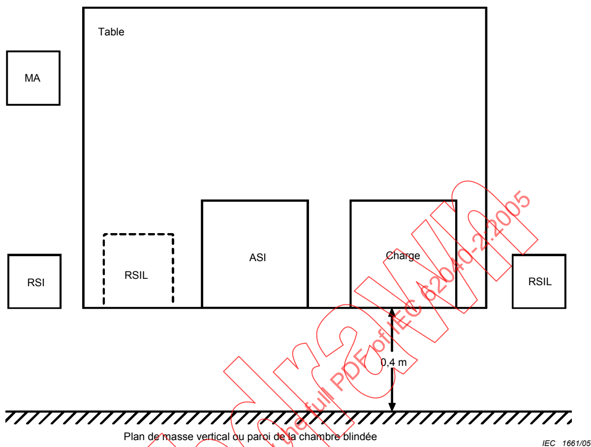
Figure A.6 – Configuration d'essai pour équipements de table (mesure des perturbations conduites) – Vue générale
