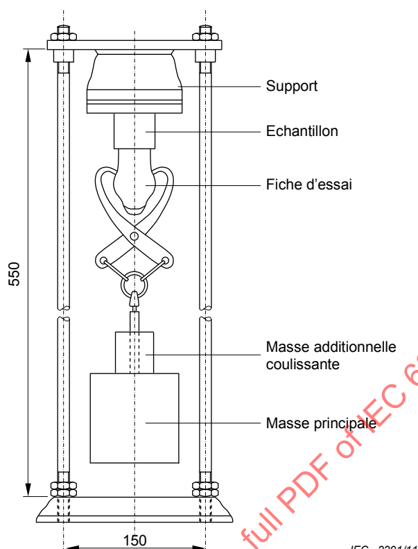
Figure 8 – Appareil de contrôle de la force d'extraction
