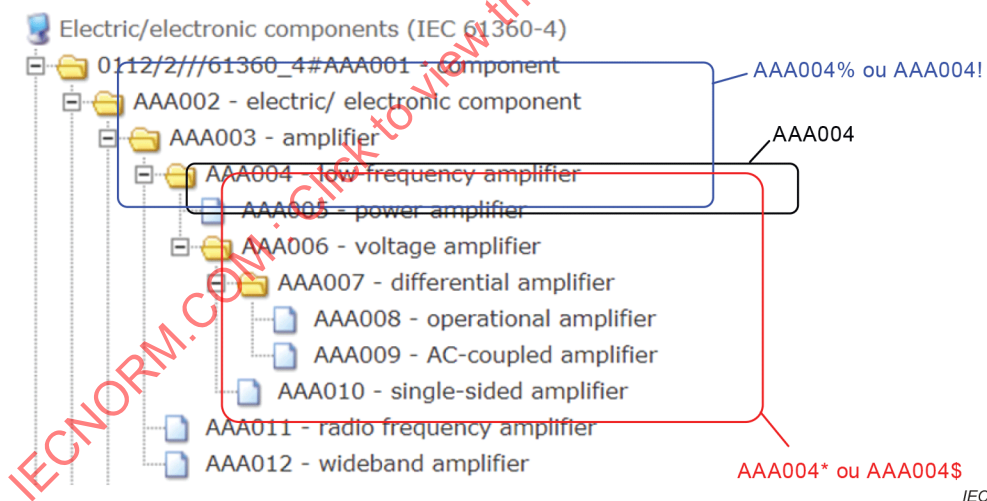
Figure 5 – Exemple de vue structurale de l'utilisation des modificateurs de domaine de recherche
