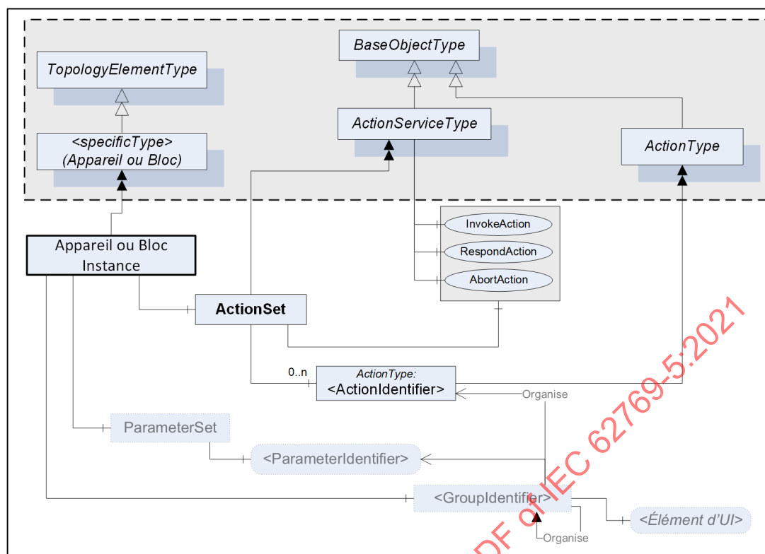
Figure 13 – Intégration des Actions au sein de TopologyElement
