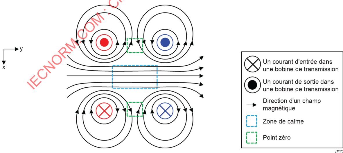
Figure 6 – Points zéro dans une zone de charge (vue de dessus)
