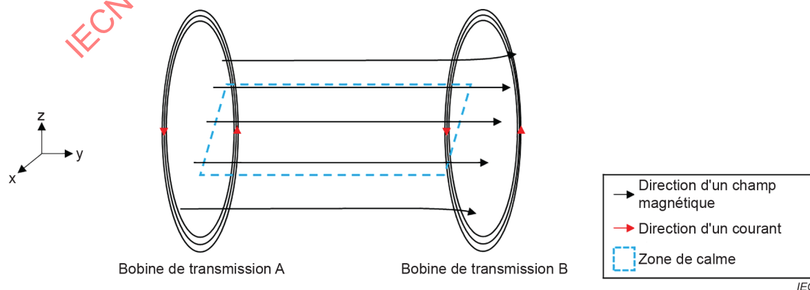
Figure 4 – Interaction entre les bobines de transmission pour générer une zone de calme
