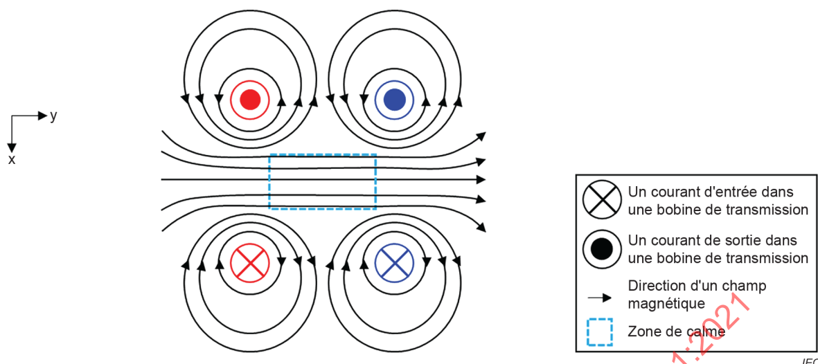
Figure 5 – Interaction entre les bobines de transmission pour générer une zone de calme (vue de dessus)
