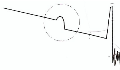
Figure 2 – Tracé d'onde typique du RDT – Puissance rétrodiffusée par rapport à la distance (km)
