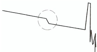
Figure 2 – Tracé d'onde typique du RDT – Puissance rétrodiffusée par rapport à la distance (km)
