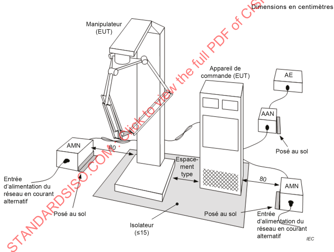
Figure 6 – Exemple de montage d'essai type pour le mesurage des perturbations conduites sur un système robotique posé au sol
