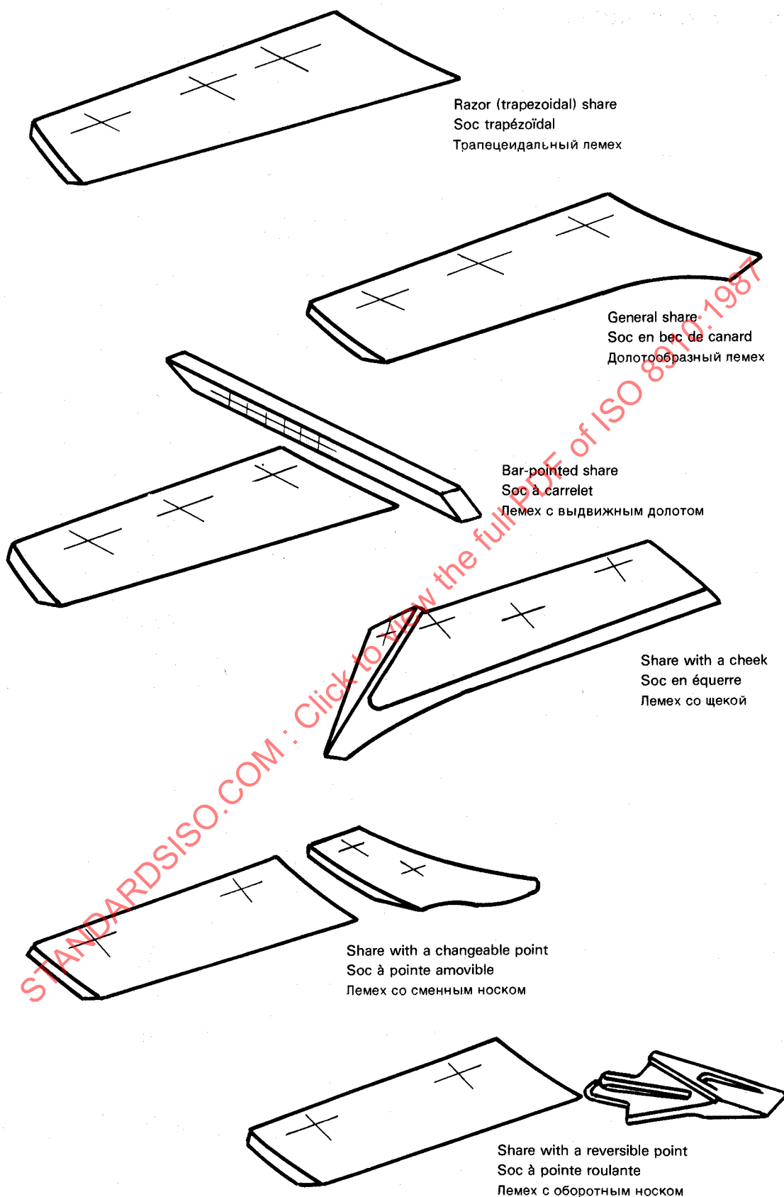
Figure 3 — Share types Figure 3 — Types de socs Рисунок 3 — Типы лемехов
