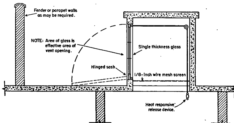
Fig. 3. Decomposition Vent.
